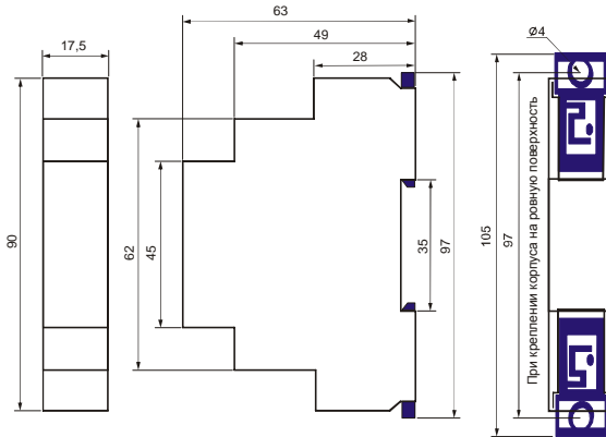
ГАБАРИТНЫЕ РАЗМЕРЫ
